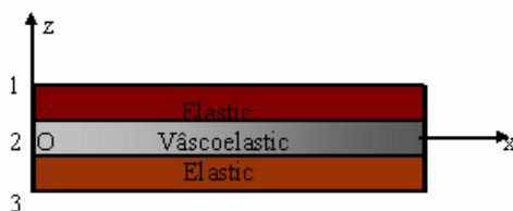
Fig.1.1 Grindă sandwich
